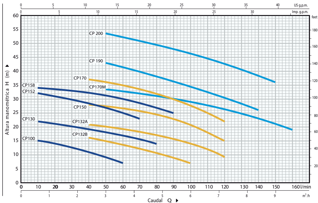
DATOS DE FUNCIONAMIENTO A n= 2900 1/min
